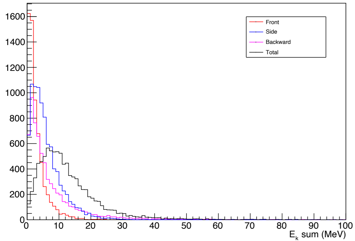
EM Standard
