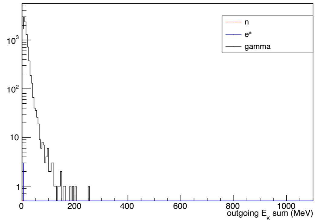
EM standard
