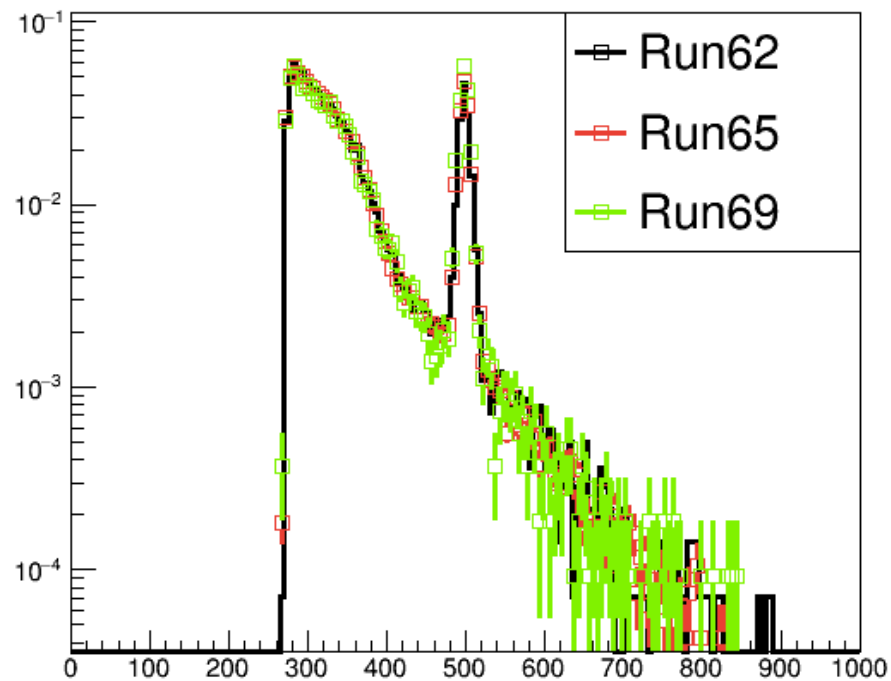
hMassOffVeto
