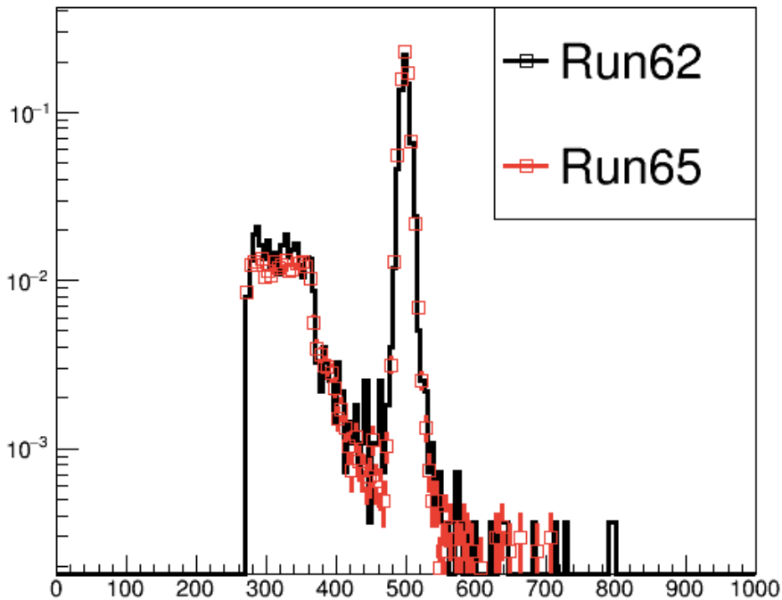
hMassSpecial
