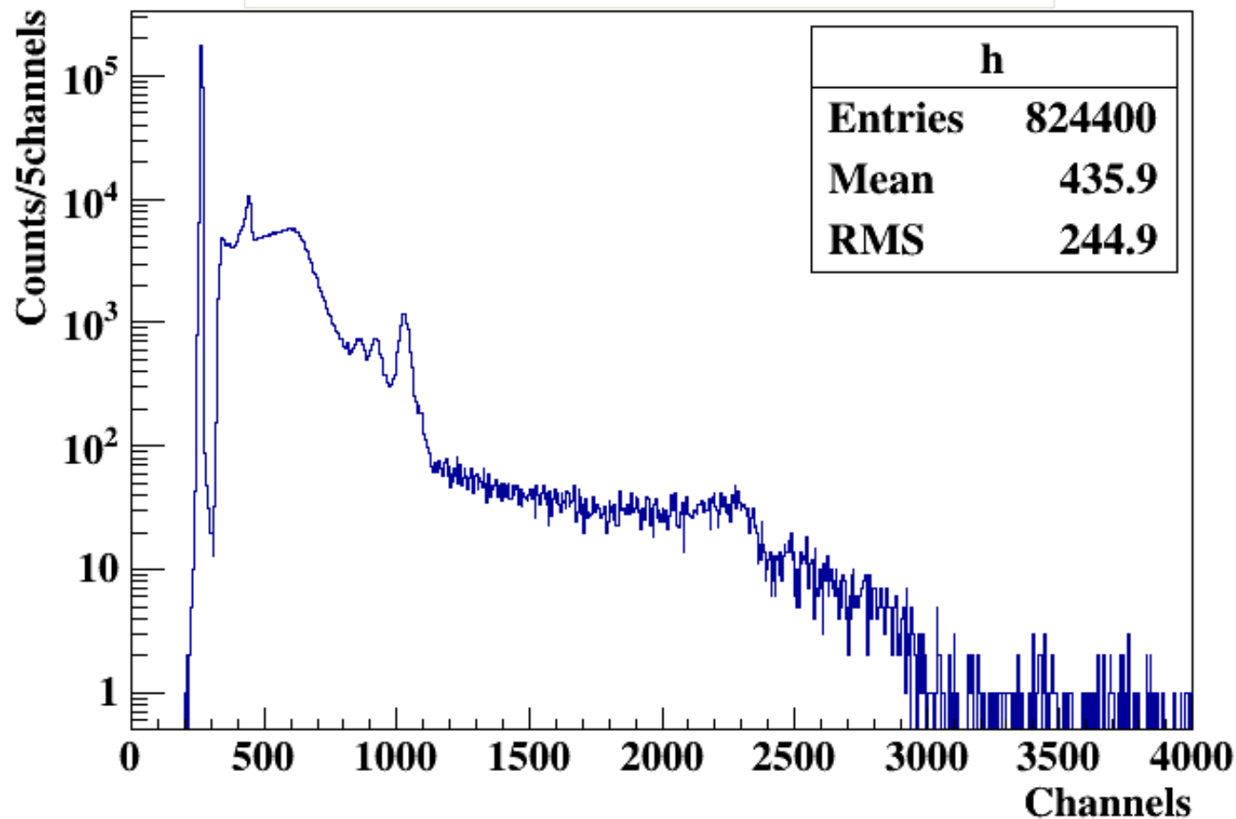
D1 Spectrum
